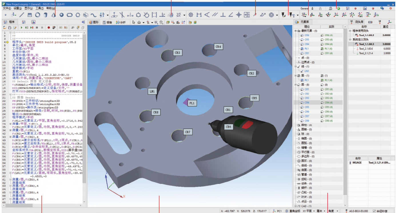
DMIS程序
